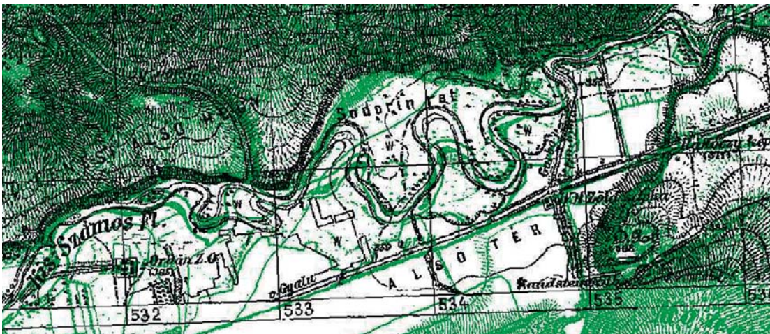
2. A Kis-Szamos mederváltozása Szászfenes (Kolozs megye) térségében a második katonai felmérés (zöld; 1859) és a harmadik katonai felmérés (fekete; 1890) között. (Kapcsolódó cikket lásd a 12. oldalon)
