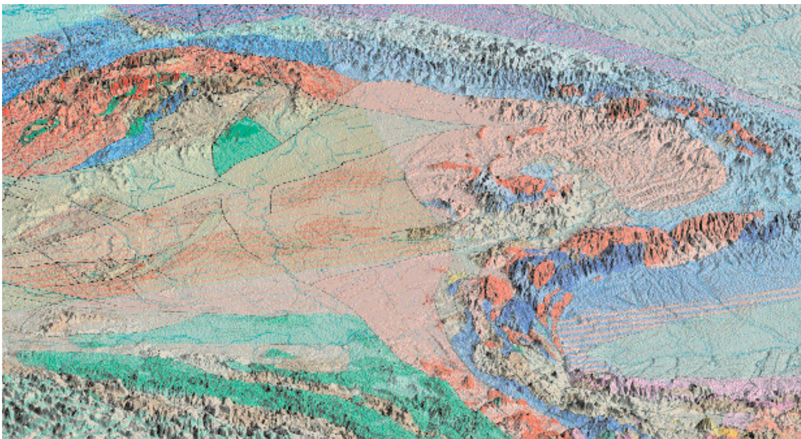
A Kárpát-Balkán-Dinári térség metamorf képződményeinek térképe (Szádeczky-Kardoss et al., 1976) és a GTOPO30 globális digitális domborzati modell (GLOBE Task Team et al., 1999) közös használatával, tízszeres magassági torzítással készített rálátási kép (cikk a 8. oldalon).
